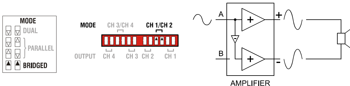
Abbildung 2.4: Betriebsart BRIDGED
